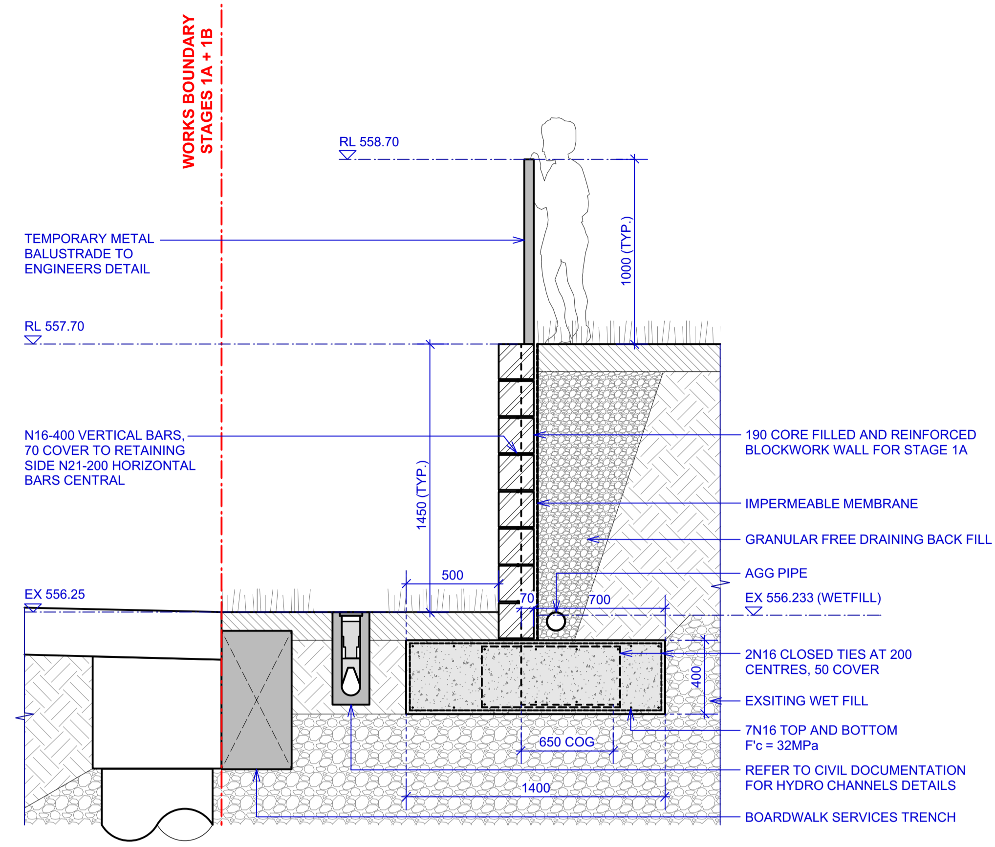
1 DETAIL SECTION - WA01.A (STAGE 1A) Scale: 1:20
